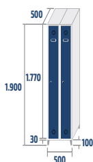
SV-25/2 COD: 42502 31kg · 0,48m 3
