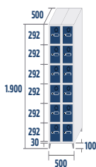
SB-25/2 COD: 42562 38,2kg · 0,48m 3
