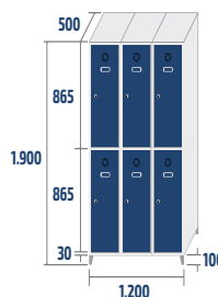
ST-40/3 COD: 44013 59kg · 1,14m 3
