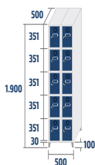
SP-25/2 COD: 42552 36,2kg · 0,48m 3
