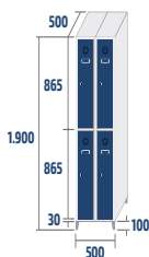
ST-25/2 COD: 42512 30,8kg · 0,48m 3
